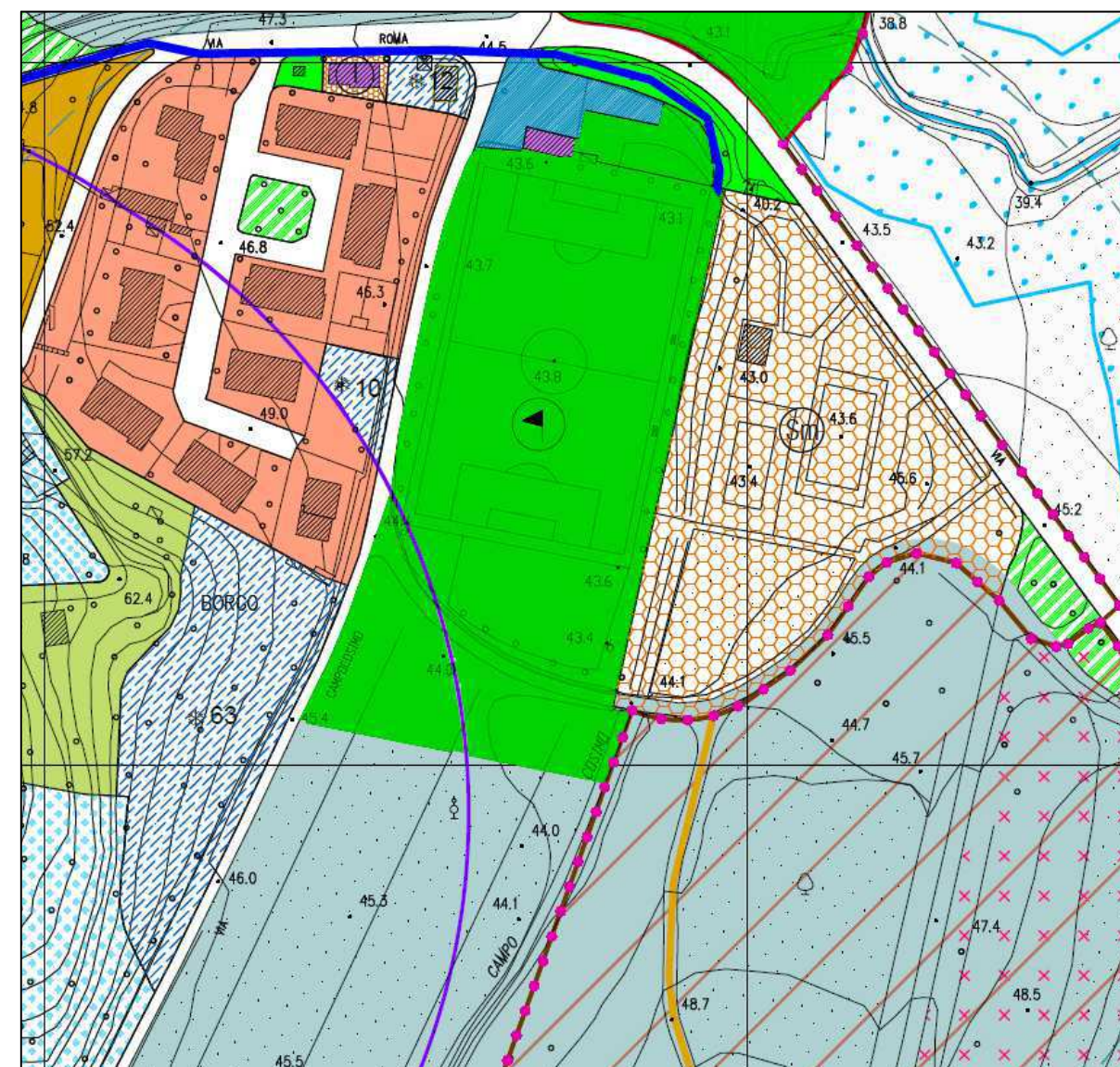
STATO IN VARIANTE sc 1:2000
