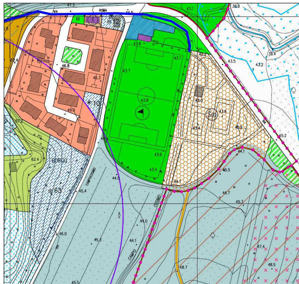
STATO ATTUALE sc 1:2000
